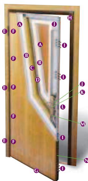
Esempio di una porta blindata certificata a2p BP 3 / Livello 5 (come da NF P 20.320)
